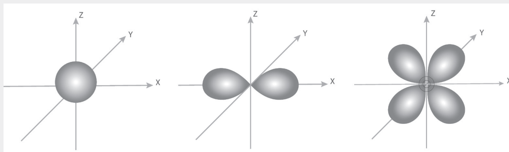
Рисунок 3. Различные формы электронного облака («геометрия» квантовой химии): 1) s-орбиталь — электронное облако в форме шара (знак круга); 2) p-орбиталь — форма гантели или двойной груши (знак бесконечности); 3) d-орбиталь — форма четырёхлепесткового цветка (знак креста).
