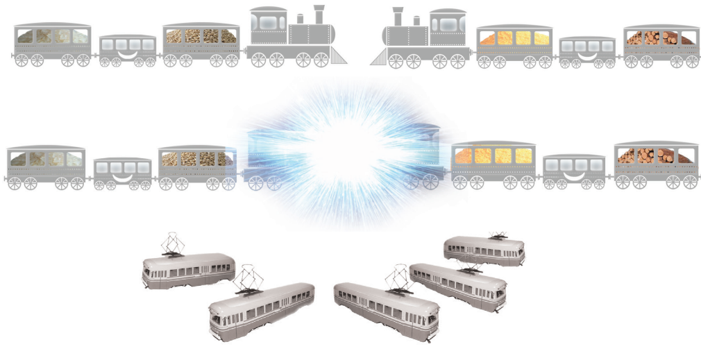
Рис.9. Ассоциативный пример столкновения двух фантомных частичек По в эзоосмической ячейке и процесса преобразования их внутреннего потенциала после прохождения эзоосмической мембраны.
