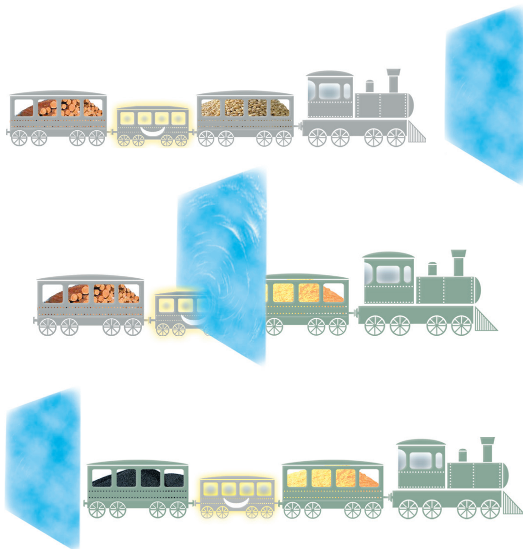
Рис. 10. Ассоциативный пример изменения внутреннего потенциала при прохождении эзоосмической мембраны.
